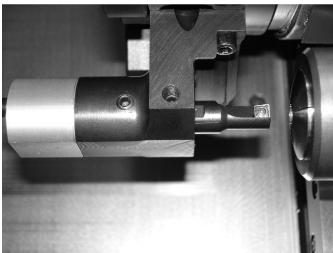
Werkzeughalter für Zylinderschaftdurchmesser mit Kühlmittelzufuhr erhältlich für \varnothing 16 mm, \varnothing 12 mm, \varnothing 10mm
