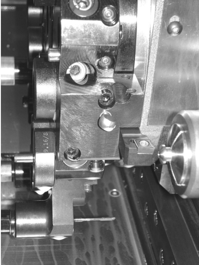
Werkzeughalter für Gegenspindel mit Kühlmitteldüse erhältlich für Vierkant 12 und Vierkant 16
