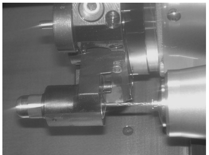
Werkzeughalter für Spannzangen mit Kühlmittelzufuhr erhältlich für 324 E, 318 E (W12), 349 E (W20)
