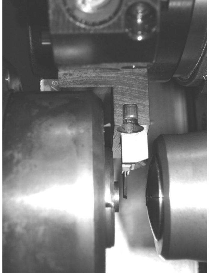
Abstechhalter Vierkant 10
